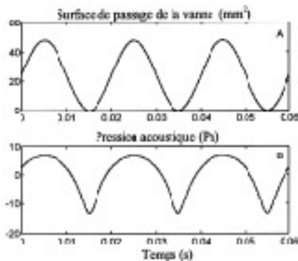
Fig.3 : Pression acoustique à la sortie de la source sonore (B), pour une modulation sinusoidale de la vanne (A).
